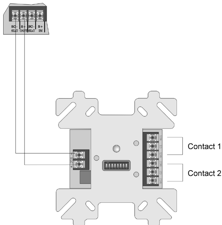
SD500-ARM Wiring
