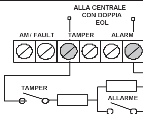
Schema di collegamento delle resistenze EOL
